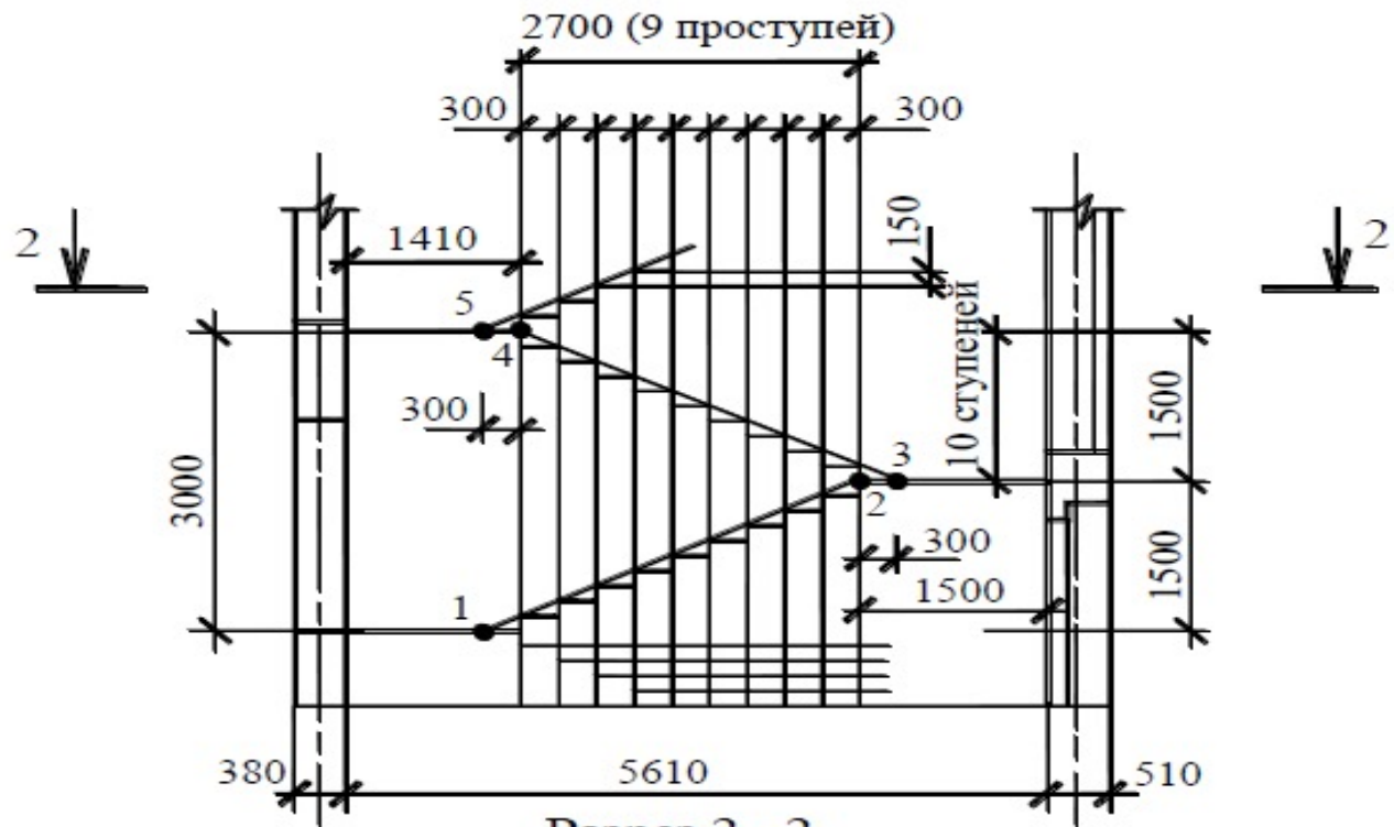
Разрез 2 - 2
